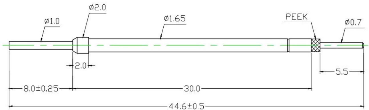
Disegno sonda di prova commutazione
