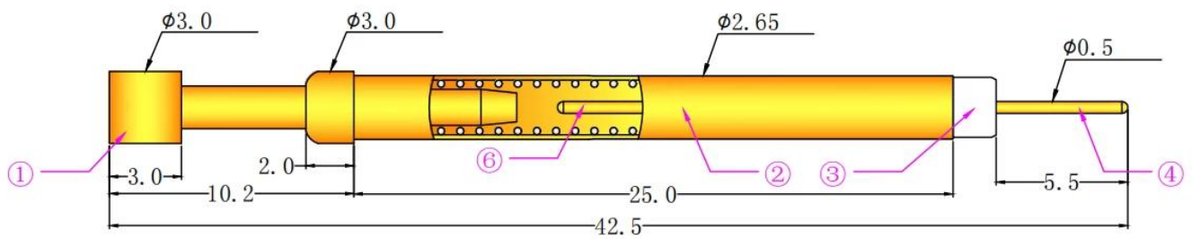
Disegno sonda di prova commutazione
