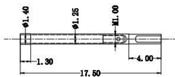
L101-套管
