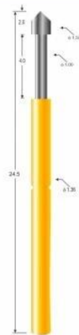
SF-P160-E
