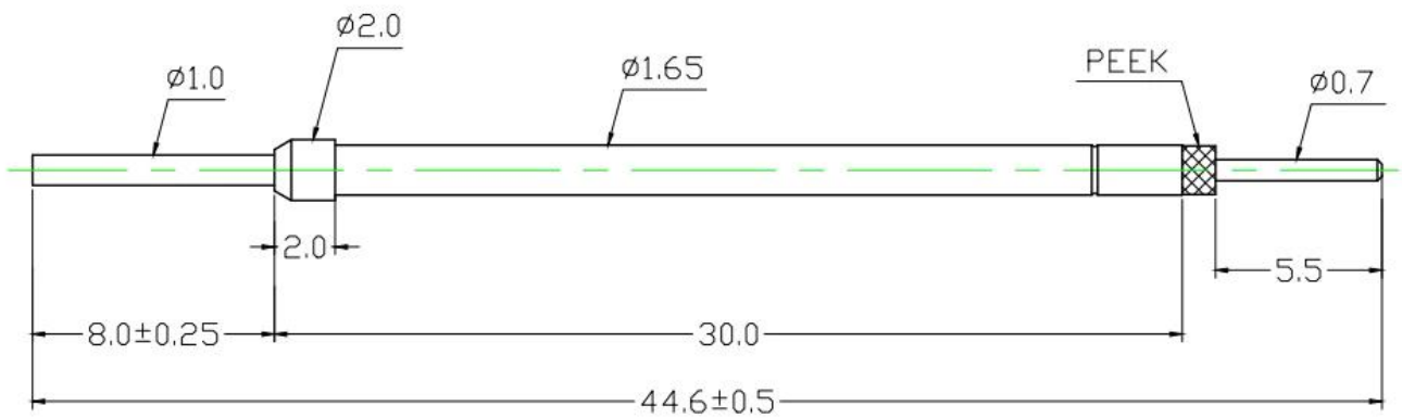
Schakelende test sonde tekening
