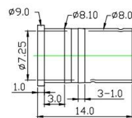
名称: SF-BR-35A大电流针ø7.2X47
