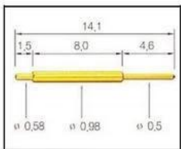
SF-P141G-098
