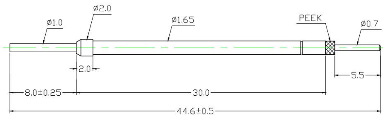
Чертеж переключающего тестового щупа
