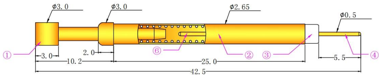
Чертеж переключающего тестового щупа
