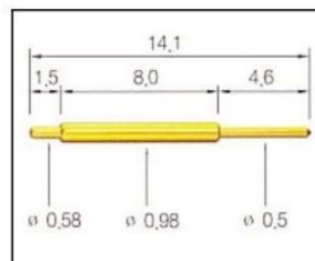
SF-P141G-098
