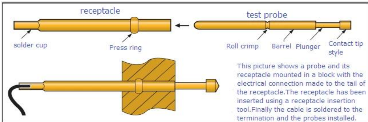
Hình ảnh sản phẩm đầu dò tiếp xúc mùa xuân
