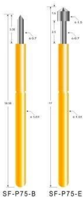
Hình ảnh sản phẩm pin đầu dò thử nghiệm PCB
